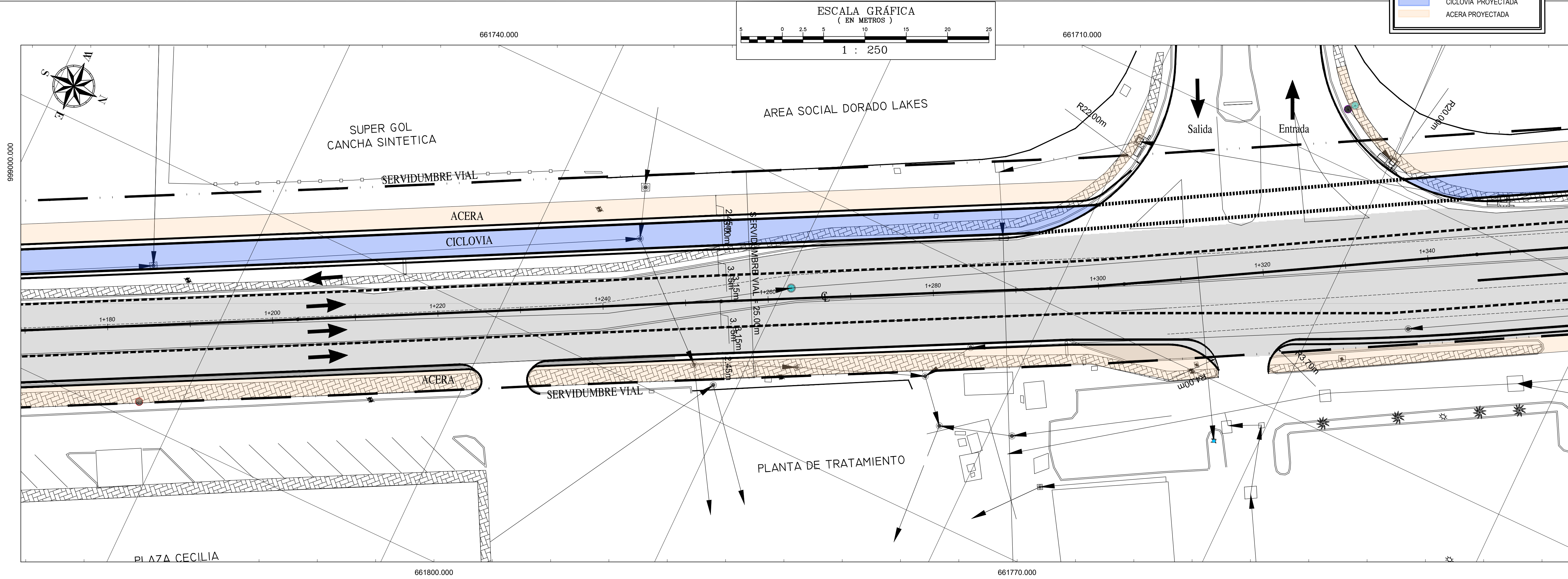
PLANTA GEOMETRICA
