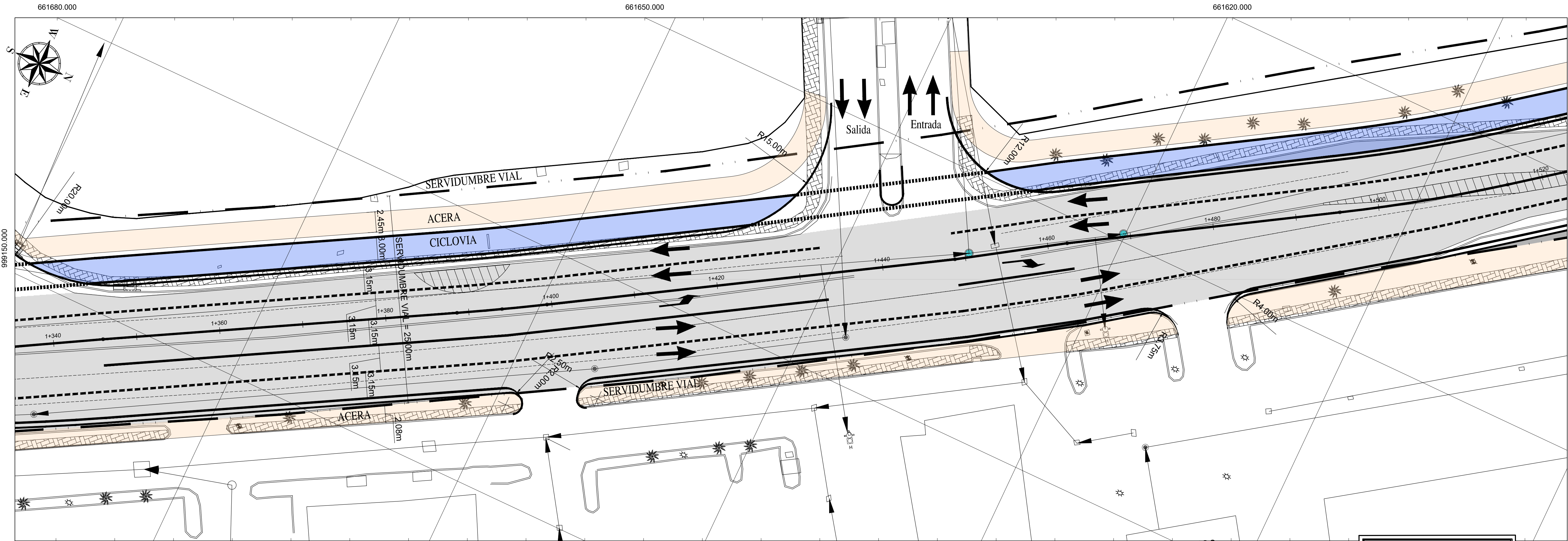
PLANTA GEOMETRICA
