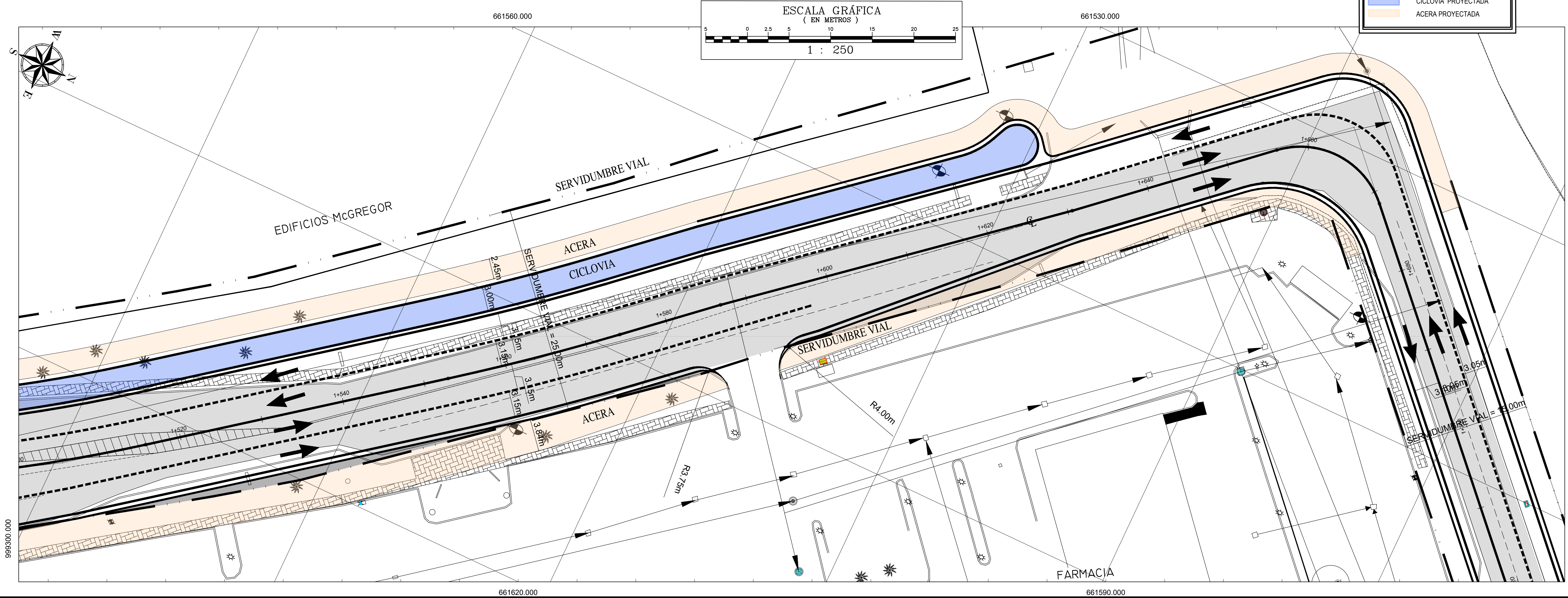
PLANTA GEOMETRICA
