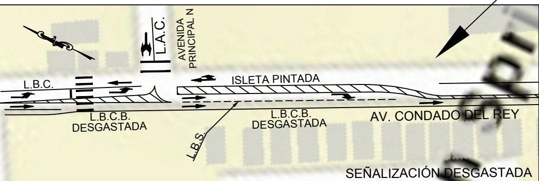
VISTA AMPLIADA DE LA SEÑALIZACIÓN HORIZONTAL EN LA INTERSECCIÓN DE LA AV. CONDADO DEL REY CON LA AV. PRINCIPAL N
