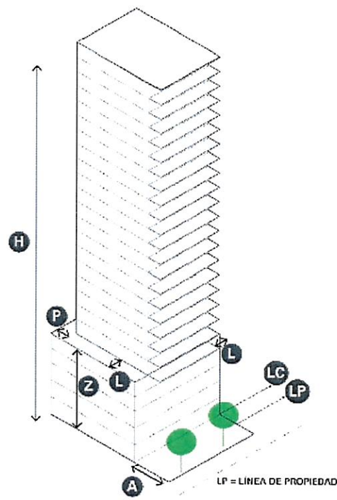
DIAGRAMA ESQUEMÁTICO
