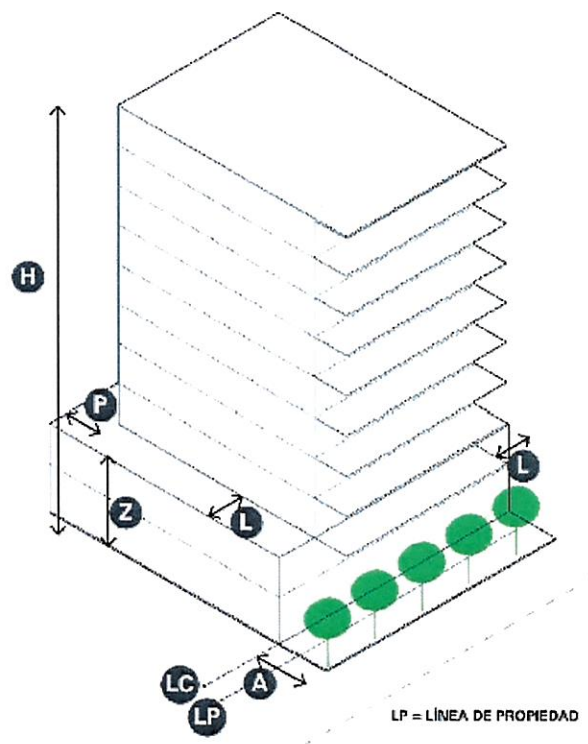
DIAGRAMA ESQUEMÁTICO
