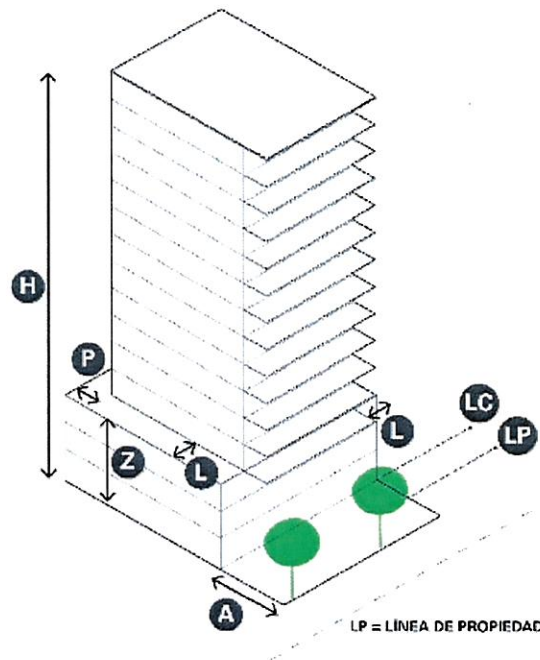
DIAGRAMA ESQUEMÁTICO
